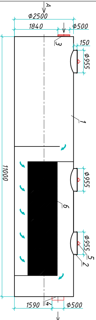
Разрез 1-1
